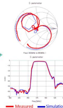
S Parameter
