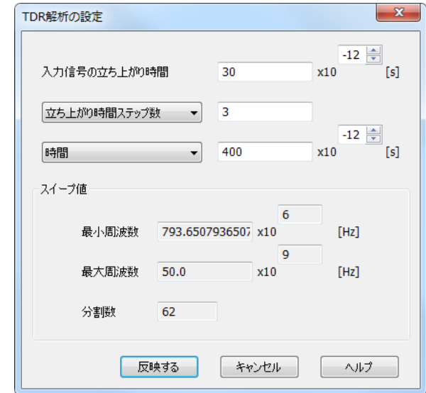
時間の設定から周波数の設定への変換
