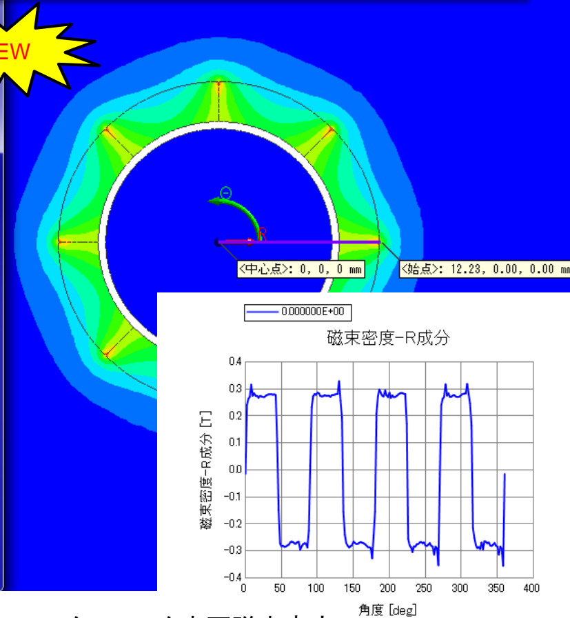
モータのロータ表面磁束密度
