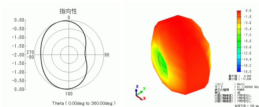
2次元指向性
