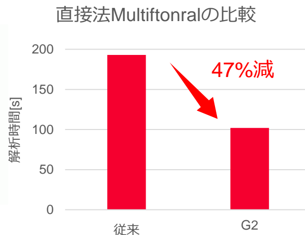
応力解析：例題 1 静解析（要素数444323）
