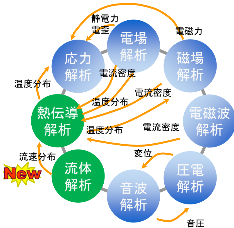
連成解析機能
