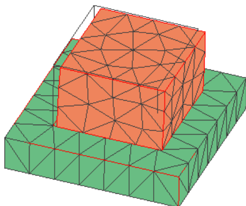
応力解析例題43 摩擦を考慮した接触解析1
