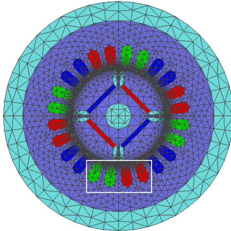
対称面でメッシュが対称
