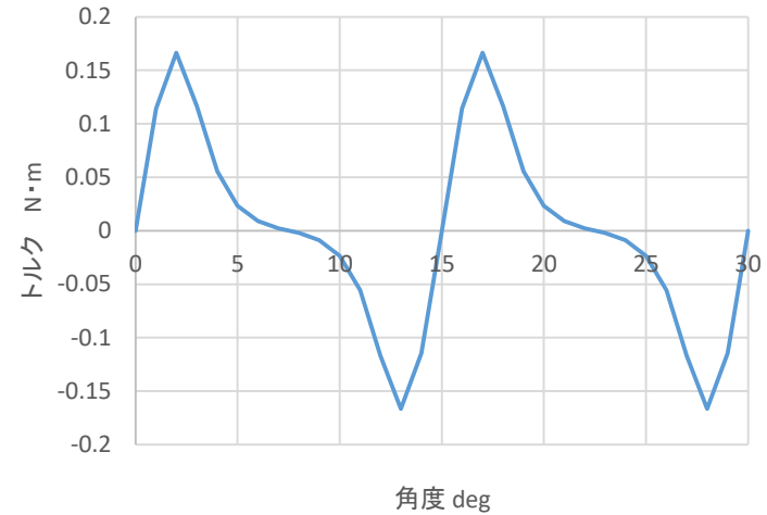
コルギングトルク
