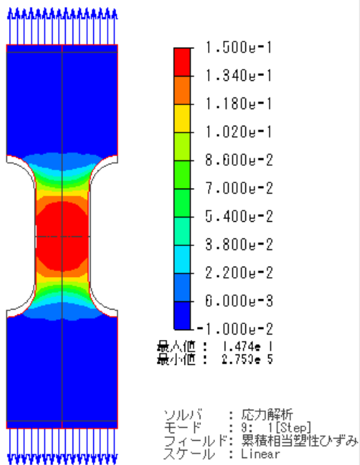
例題 4 0 弾塑性マルチリニア材料の変形解析
