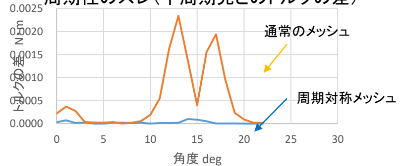
周期性のズレ(半周期先とのトルクの差)
