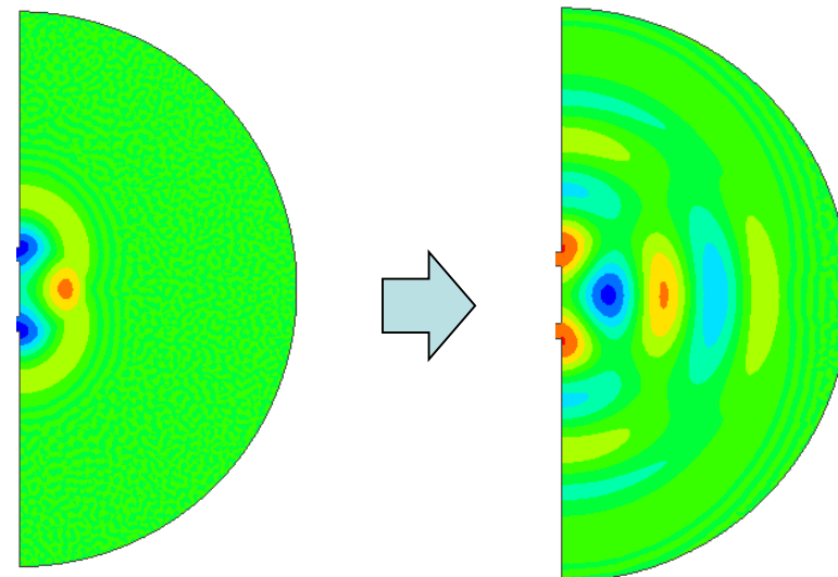
音波解析例題3: 音波が伝搬する過程
