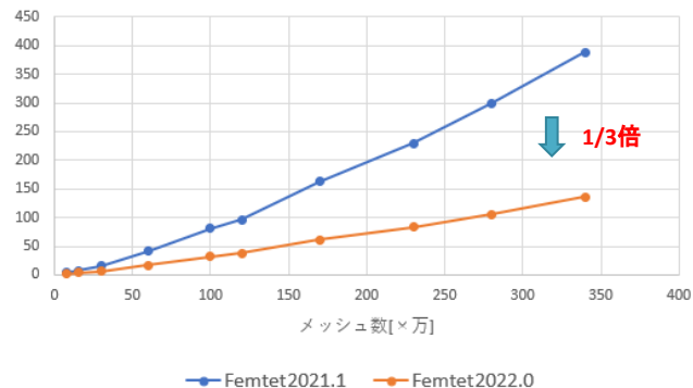
消費メモリ [GB]
