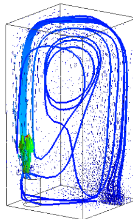
流速と流線
